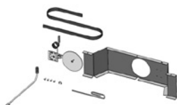
Vanne thermostatique d'entrée air de combustion Thermostatische controleklep toevoer verbrandingslucht
