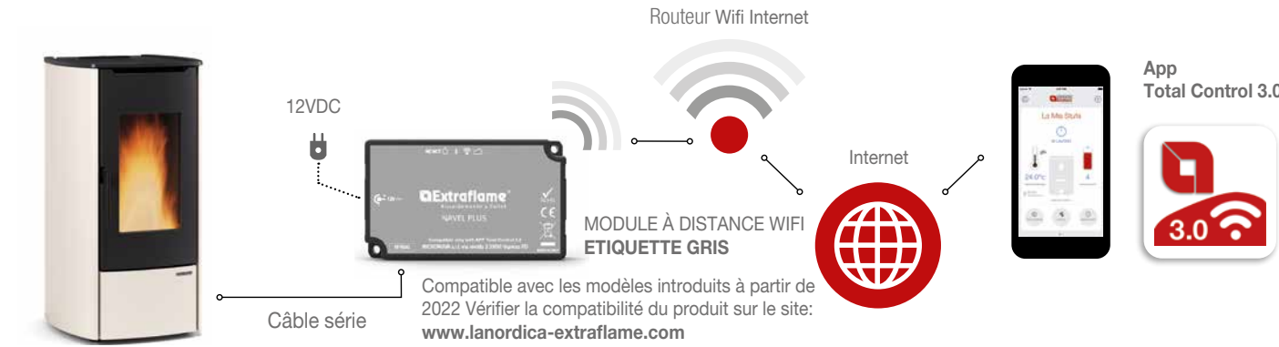
Schéma Module à distance Wifi - ETIQUETTE GRIS (C)
