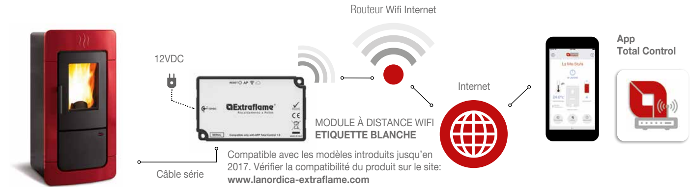
Schéma Module à distance Wifi - ETIQUETTE BLANCHE (A)
