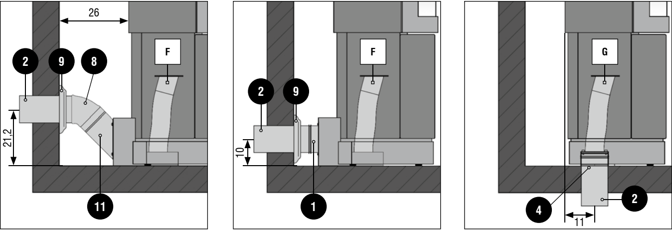
Jena B.11 Anschlussmaße für Wand- und Bodenanschluss · Connection dimensions for Jena B.11 wall and bottom connection · Dimensions du raccord pour Jena B.11 en cas de raccordement au mur et au sol · Dimensioni di collegamento per Jena B.11 per il collegamento alla parete e al pavimento · Aansluitingsmaten voor Jena B.11 wandaansluiting of vloeraansluiting
