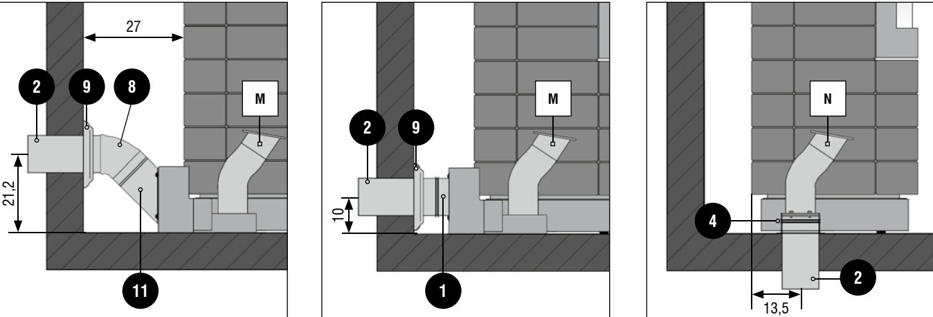
Lisboa C.15 Anschlussmaße für Wand- und Bodenanschluss · Connection dimensions for Lisboa C.15 wall and bottom connection · Dimensions du raccord pour Lisboa C.15 en cas de raccordement au mur et au sol · Dimensioni di collegamento per Lisboa C.15 per il collegamento alla parete e al pavimento · Aansluitingsmaten voor Lisboa C.15 wandaansluiting of vloeraansluiting
