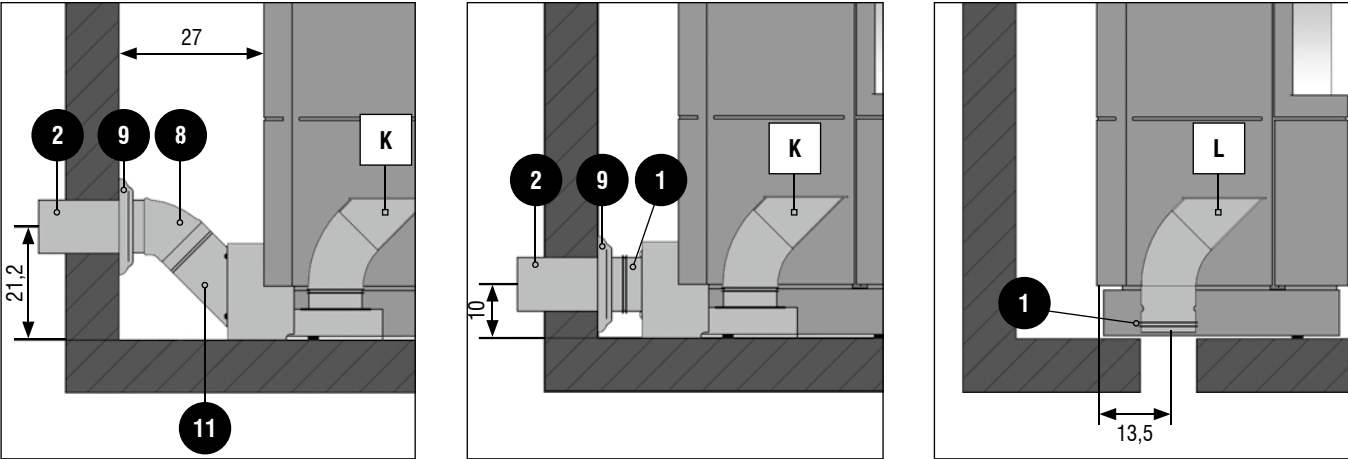
Lima / Sila / Sila Plus Anschlussmaße für Wand- und Bodenanschluss · Connection dimensions for Lima C.16 / Sila / Sila Plus wall and bottom connection · Dimensions du raccord pour Lima C.16 / Sila / Sila Plus en cas de raccordement au mur et au sol · Dimensioni di collegamento per Lima C.16 / Sila / Sila Plus per il collegamento alla parete e al pavimento · Aansluitingsmaten voor Lima C.16 / Sila / Sila Plus wandaansluiting of vloeraansluiting
