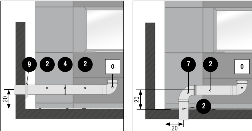
Padua 160 / 185 mit Regal Anschlussmaße für für Wand- und Bodenanschluss* · Connection dimensions for Padua 160/185 with wood box wall and bottom connection* · Dimensions du raccord pour Padua 160/185 avec woodbox en cas de raccordement au mur et au sol* · Dimensioni di collegamento per Padua 160/185 con cassetta per il collegamento alla parete e al pavimento* · Aansluitingsmaten voor Padua 160/185 met houtopslag mod wandaansluiting of vloeraansluiting*
