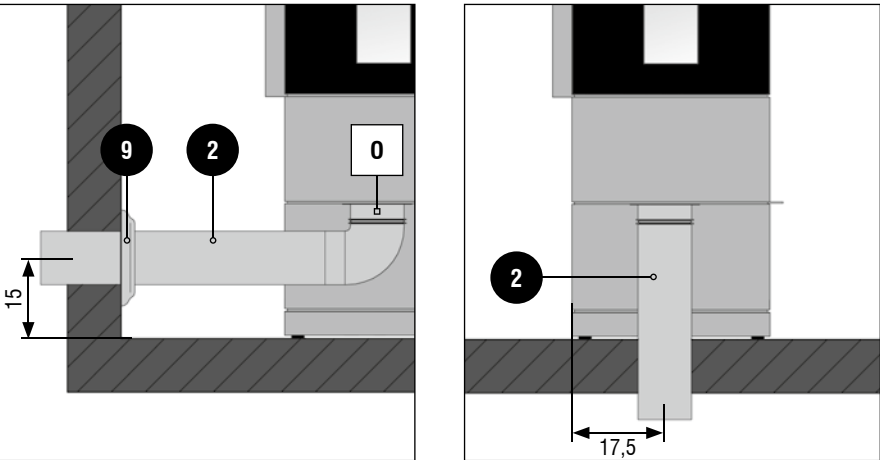
Sendai 135 / 155 Anschlussmaße für Wand- und Bodenanschluss · Connection dimensions for Sendai 135/155 wall and bottom connection · Dimensions du raccord pour Sendai 135/155 en cas de raccordement au mur et au sol · Dimensioni di collegamento per Sendai 135/155 per il collegamento alla parete e al pavimento · Aansluitingsmaten voor Sendai 135/155 wandaansluiting of vloeraansluiting
