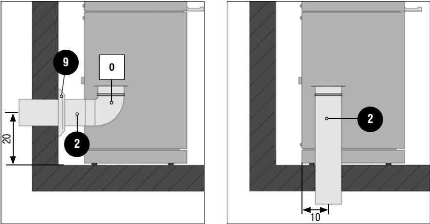
Padua 160 / 185 Anschlussmaße für Wand- und Bodenanschluss · Connection dimensions for Padua 160/185 wall and bottom connection · Dimensions du raccord pour Padua 160/185 en cas de raccordement au mur et au sol · Dimensioni di collegamento per Padua 160/185 per il collegamento alla parete e al pavimento · Aansluitingsmaten voor Padua 160/185 wandaansluiting of vloeraansluiting
