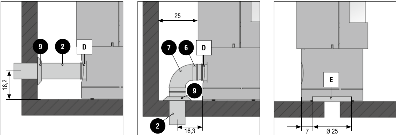
Delhi 124 Anschlussmaße für bei Wand- und Bodenanschluss · Connection dimensions for Delhi 124 wall and bottom connection · Dimensions du raccord pour Delhi 124 en cas de raccordement au mur et au sol · Dimensioni di collegamento per Delhi 124 per il collegamento alla parete e al pavimento · Aansluitingsmaten voor Delhi 124 wandaansluiting of vloeraansluiting
