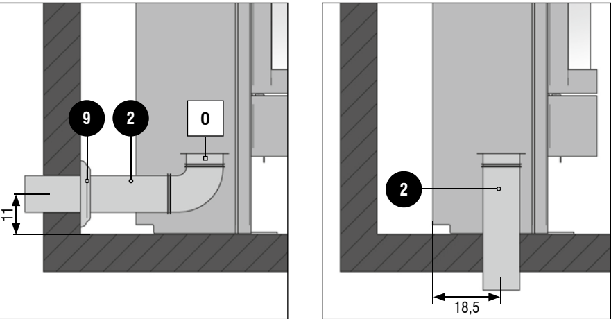
Luno B.13 Anschlussmaße für Wand- und Bodenanschluss · Connection dimensions for Luno B.13 wall and bottom connection · Dimensions du raccord pour Luno B.13 en cas de raccordement au mur et au sol · Dimensioni di collegamento per Luno B.13 per il collegamento alla parete e al pavimento · Aansluitingsmaten voor Luno B.13 wandaansluiting of vloeraansluiting
