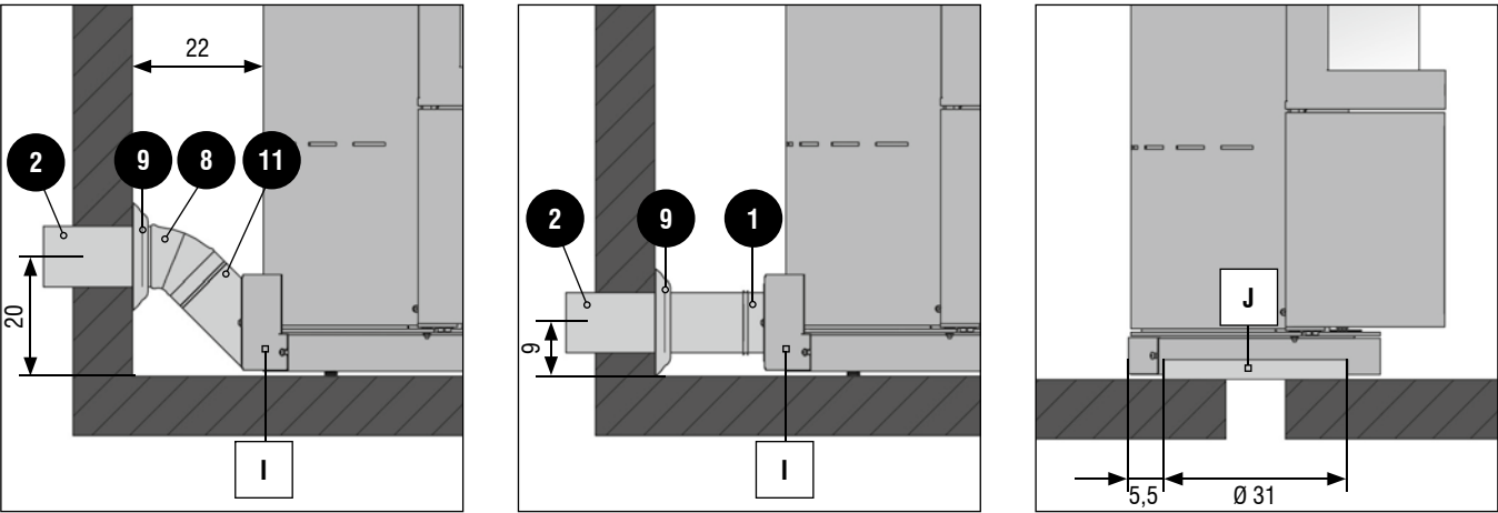
Lagos Anschlussmaße für Wand und Bodenanschluss · Connection dimensions for Lagos wall and bottom connection · Dimensions du raccord pour Lagos en cas de raccordement au mur et au sol · Dimensioni di collegamento Lagos per il collegamento alla parete e al pavimento · Aansluitingsmaten voor Lagos wandaansluiting of vloeraansluiting
