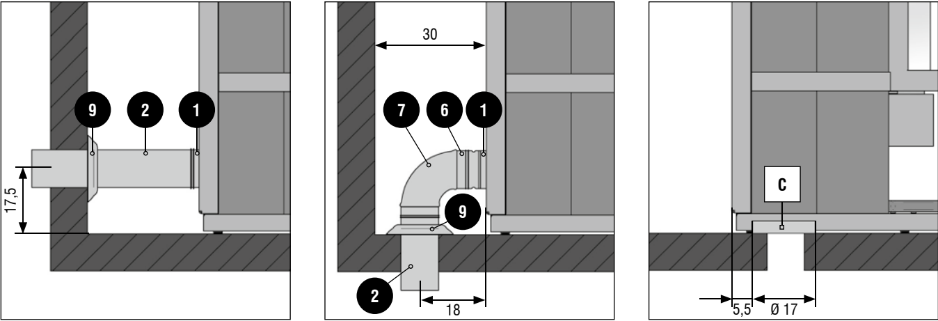
Delhi 114 Anschlussmaße für Wand- und Bodenanschluss · Connection dimensions for Delhi 114 wall and bottom connection · Dimensions du raccord pour Delhi 114 en cas de raccordement au mur et au sol · Dimensioni di collegamento per Delhi 114 per il collegamento alla parete e al pavimento · Aansluitingsmaten voor Delhi 114 wandaansluiting of vloeraansluiting
