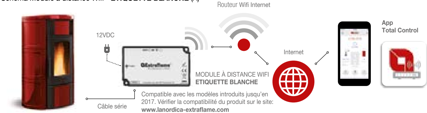
Schéma Module à distance Wifi - ETIQUETTE BLANCHE (A)
