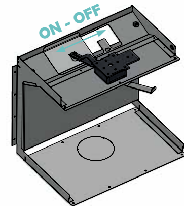
PRISE D AIR MANUEL ON/ OFF / BUITENLUCHTTOEVOER MANUEEL ON/ OFF
